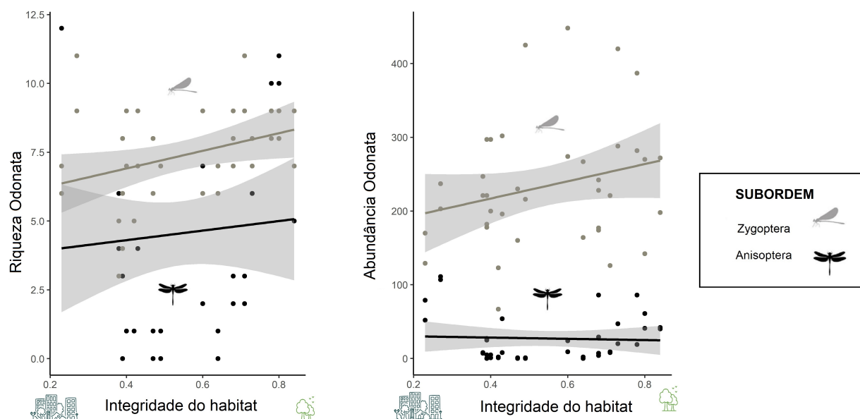
Figura 2. Relação entre a integridade do habitat e a riqueza e abundância de espécies de odonatos. A área sombreada indica os intervalos de confiança de 95%.
